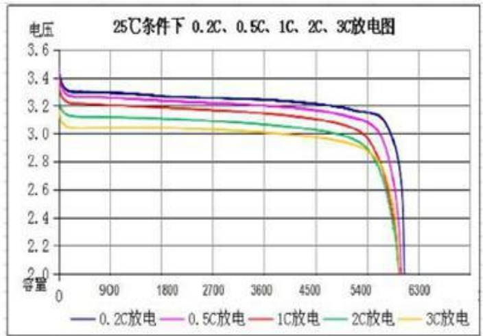
放电曲线图 Diploid discharge curve
